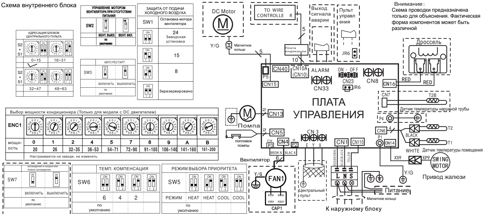
Схема внутреннего блока
